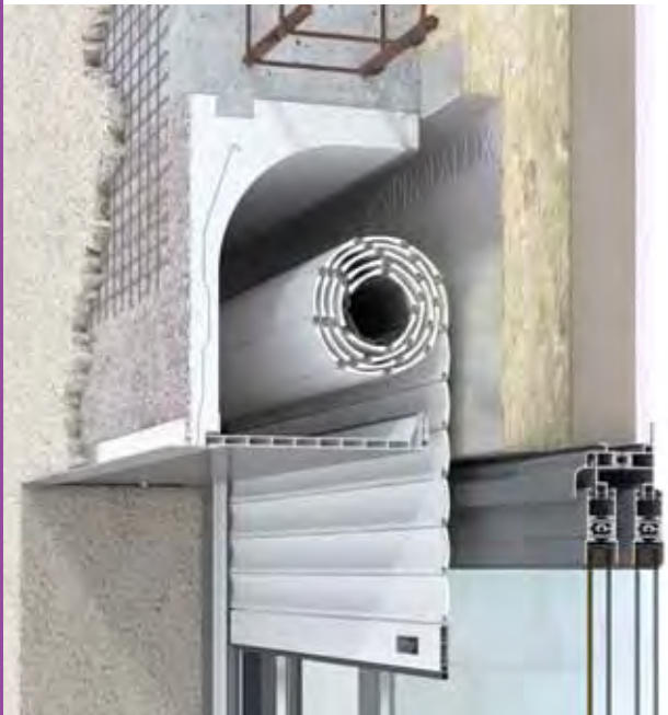
[Enroulement extérieur]
