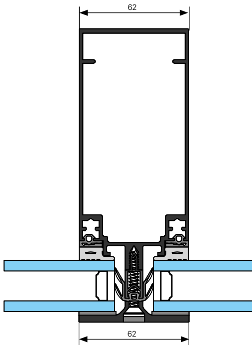
Trame horizontale suivant nouvelle réglementation en vigueur
