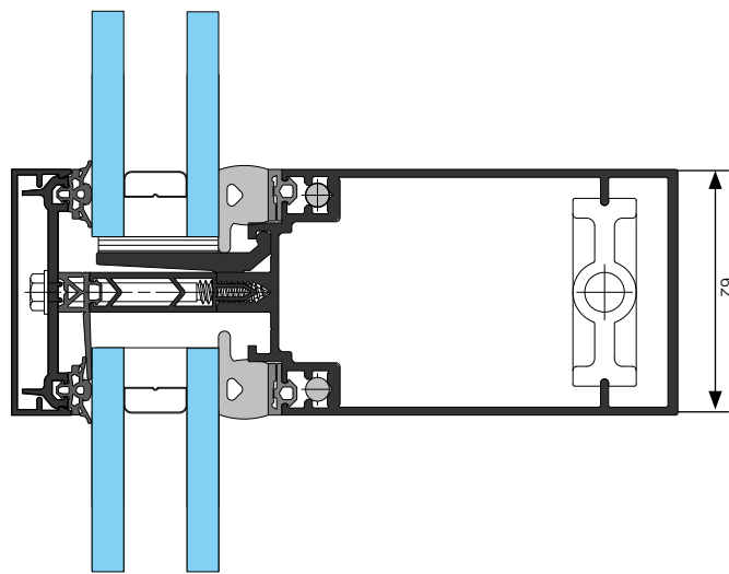
Serreur filant
