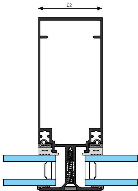
Serreur capot plat
