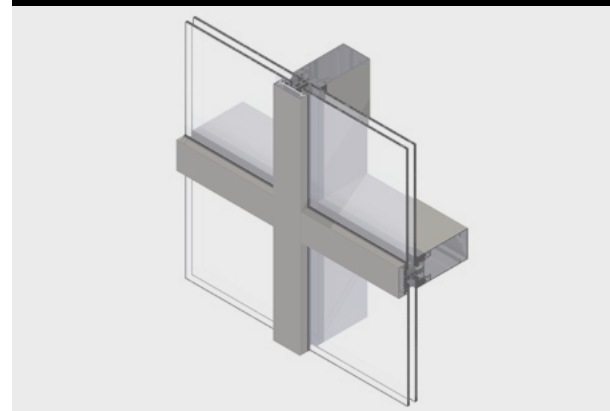
SPINAL GRILLE APPARENTE
