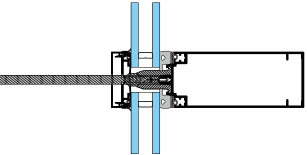
Façade SPINAL avec intégration de la patte support
