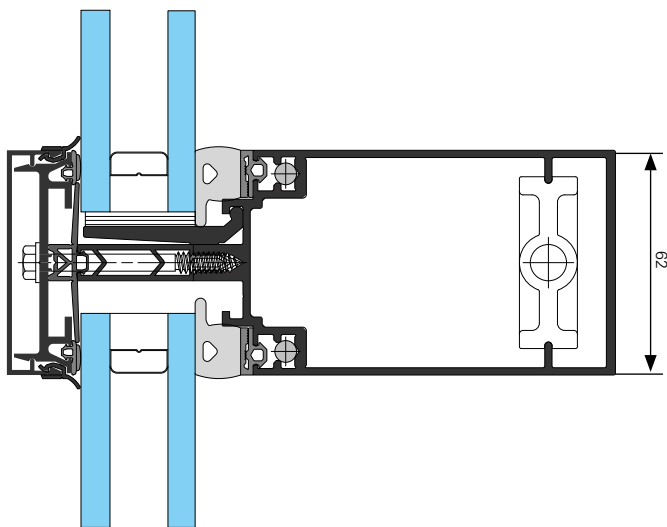
Serreur ponctuel
