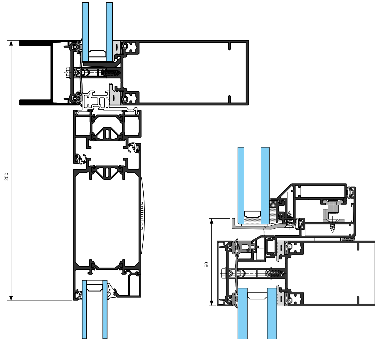
Intégration porte TITANE 65*
