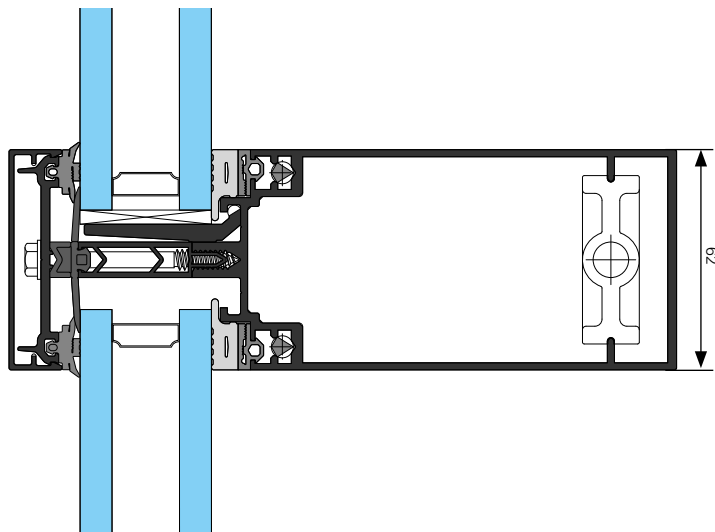
Drainage caché sur joint central
