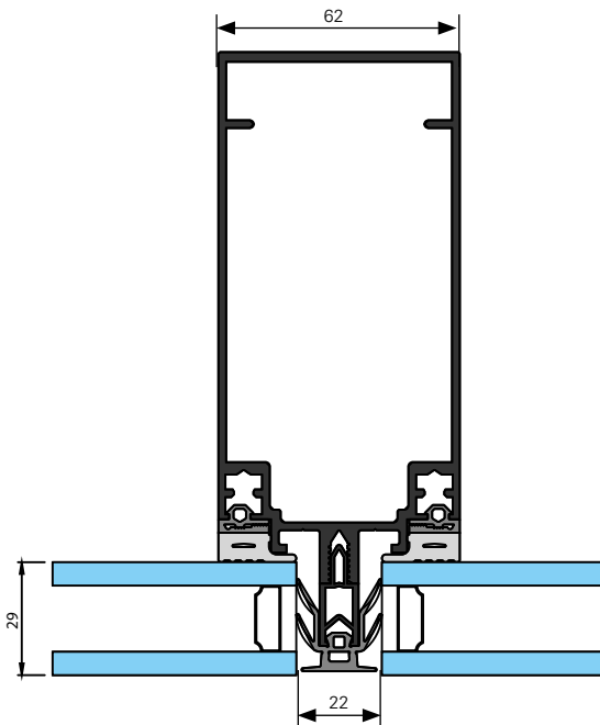
Trame horizontale
